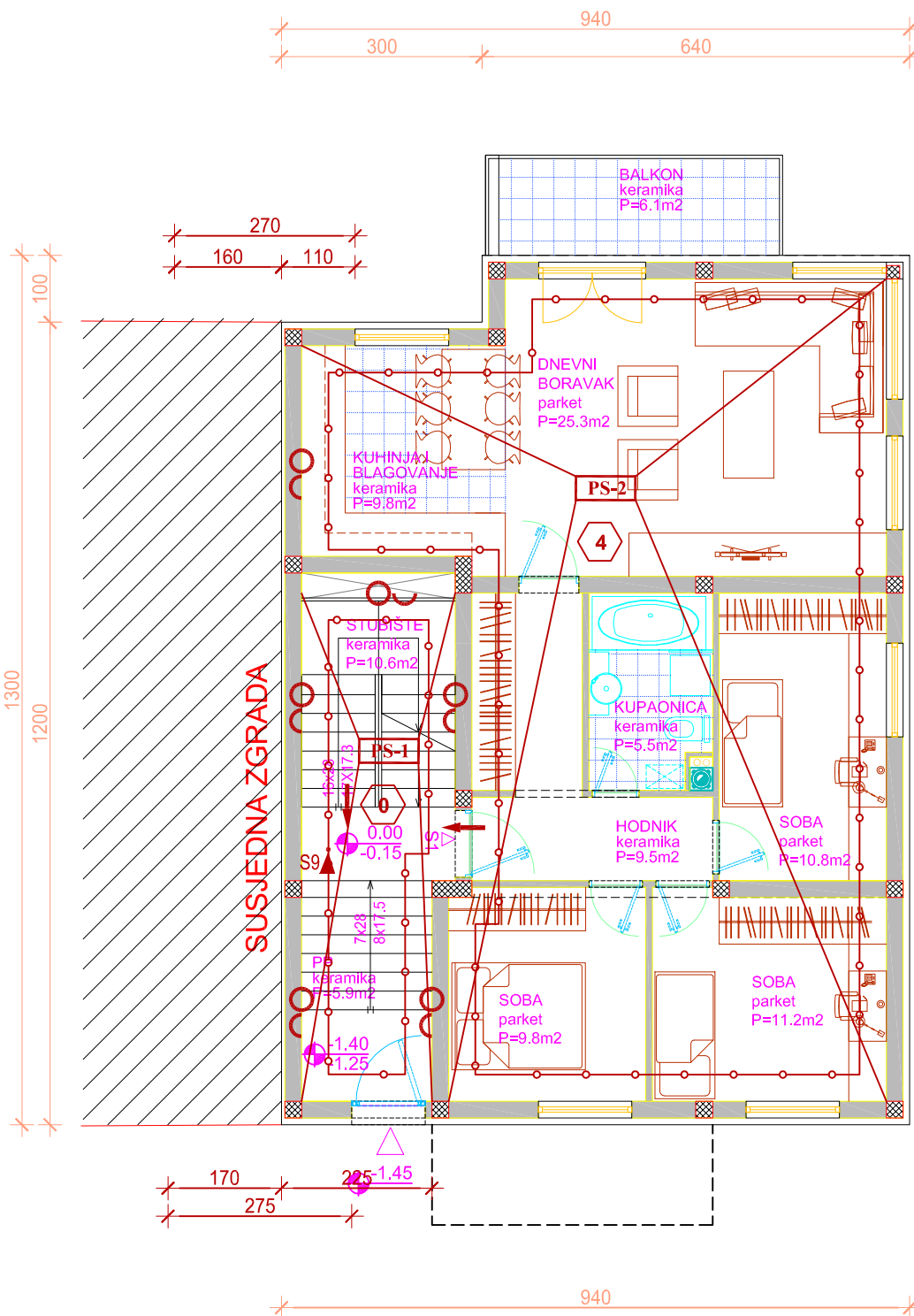
TLOCRT PRIZEMLJA
